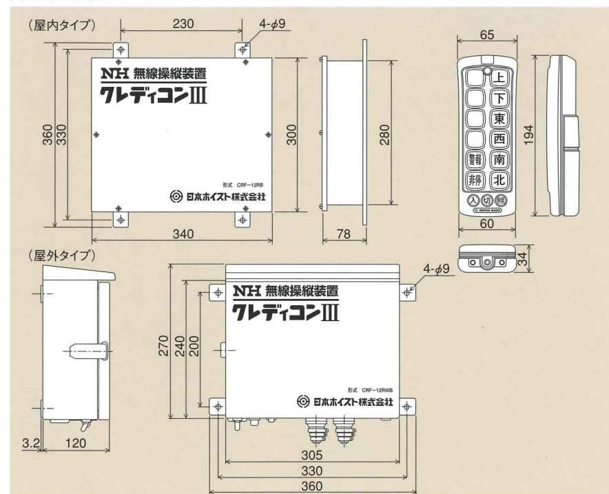
外形寸法図
