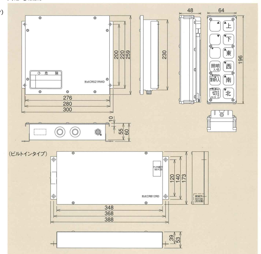
外形寸法図
